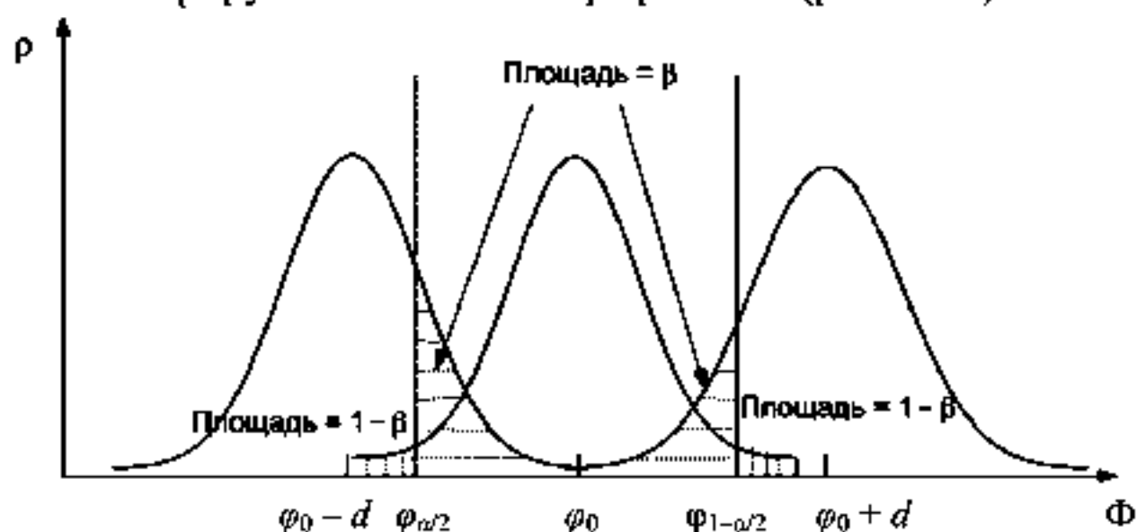
Рис. 10.3. Определение ошибки первого и второго рода при проверке гипотез
