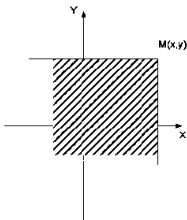
Рис. 5.1. Функция распределения двумерной СВ
