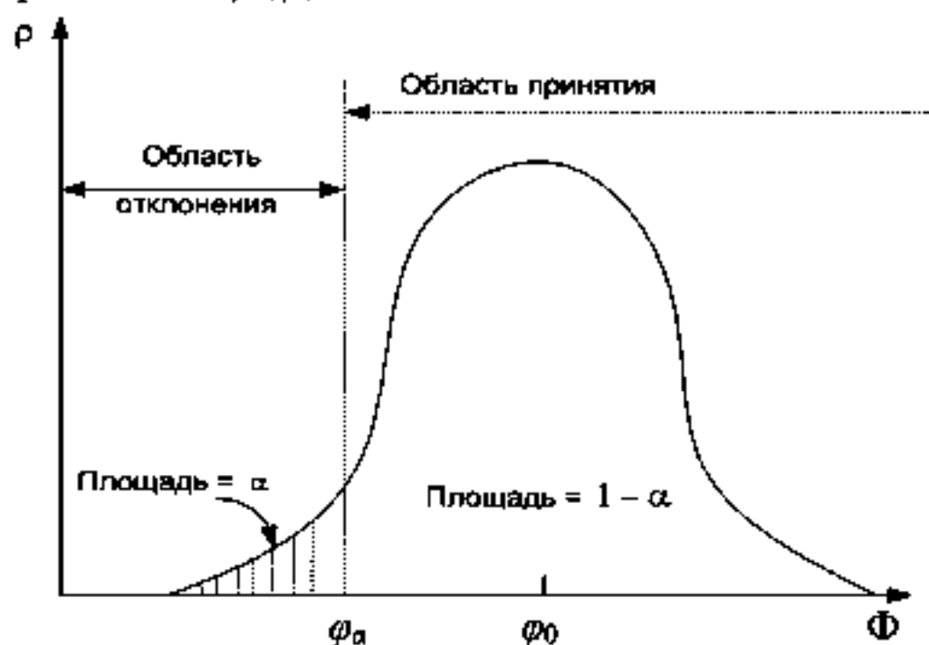
Рис. 10.2. Область принятия и отклонения гипотезы (односторонний критерий)
