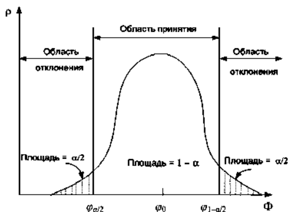
Рис. 10.1. Область принятия и отклонения гипотезы (двусторонний критерий)
