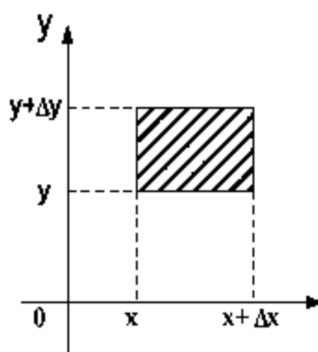
Рис. 5.3. Вероятность попадания в прямоугольник
