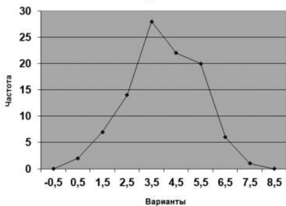
Рис. 8.2. Полигон
