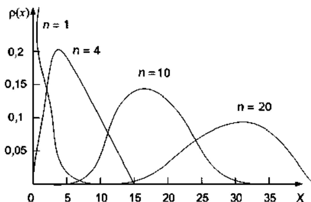
Рис. 6.4. Распределение «хи-квадрат»
