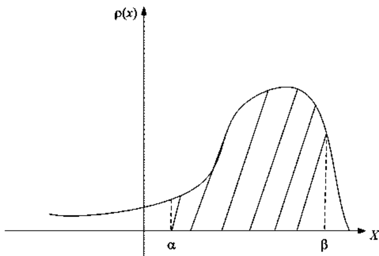
Рис. 4.3. Вероятность попадания на интервал
