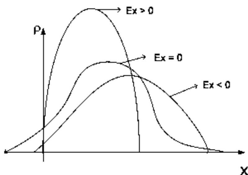
Рис. 4.8. Характеристика островершинности распределений
