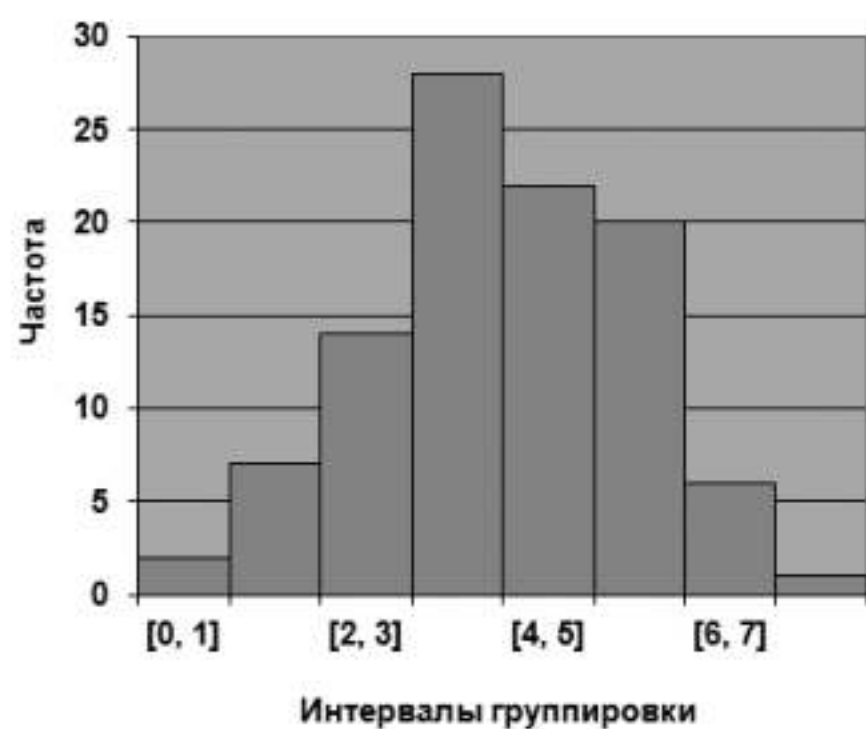
Рис. 8.1. Гистограмма частот
