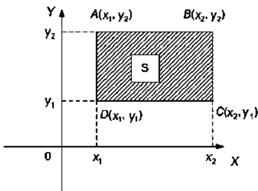
Рис. 5.2. Вероятность попадания в прямоугольник
