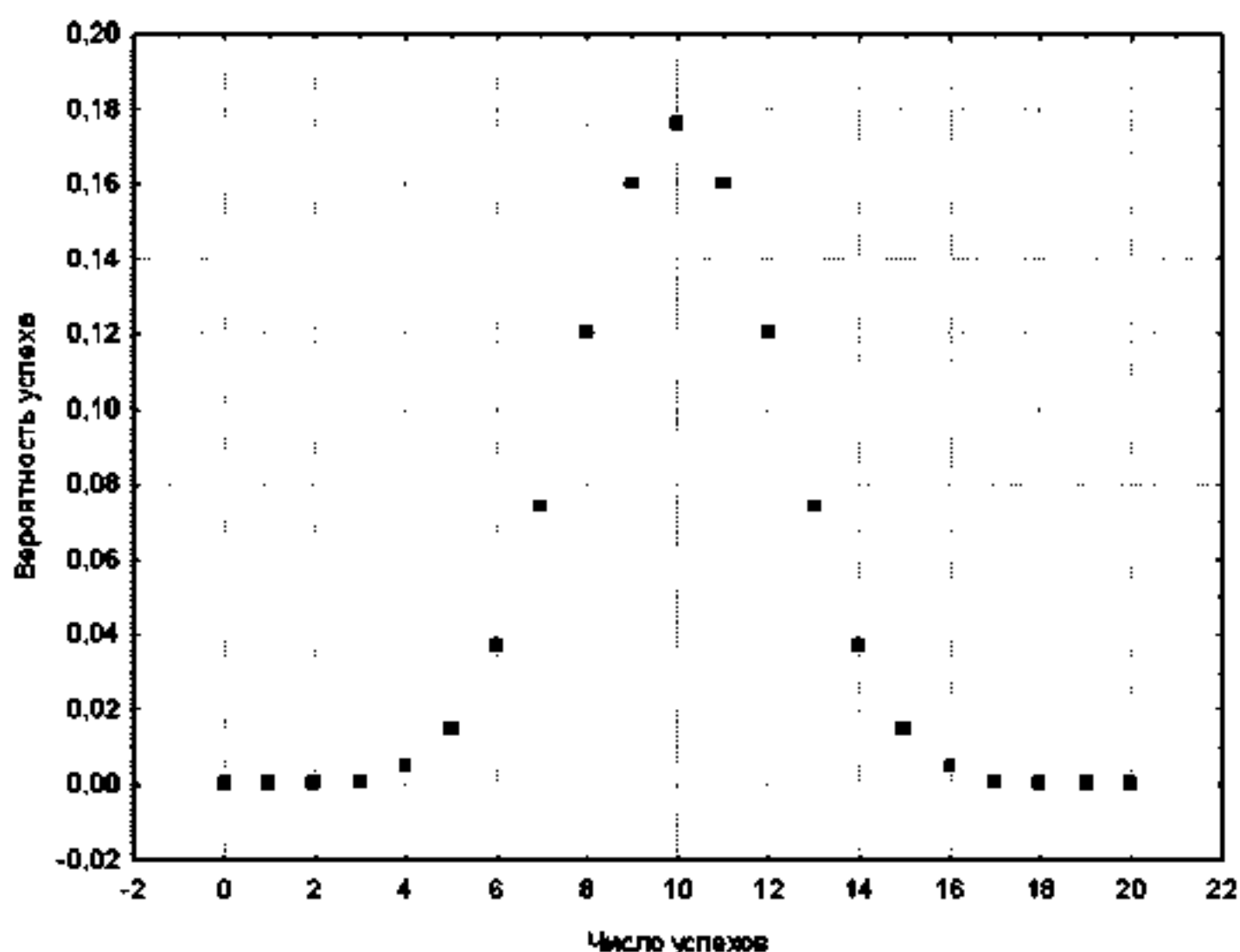
Рис. 3.1. График вероятностей биномиального распределения ( p = 0,5 ; n = 20 )
