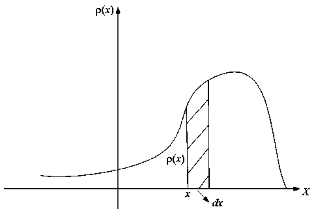
Рис. 4.2. Вероятность попадания на элементарный интервал
