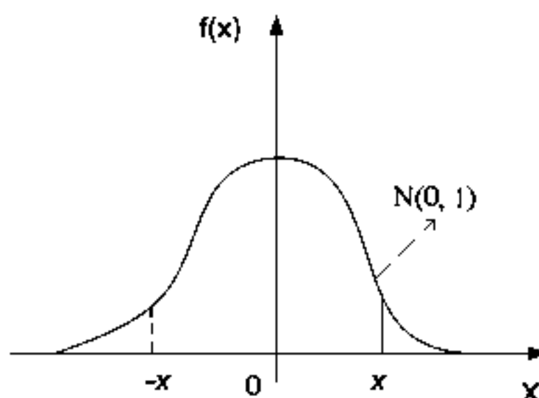
Рис. 6.2. Стандартное распределение
