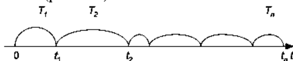
Рис. 11.3. Ординарный поток событий
