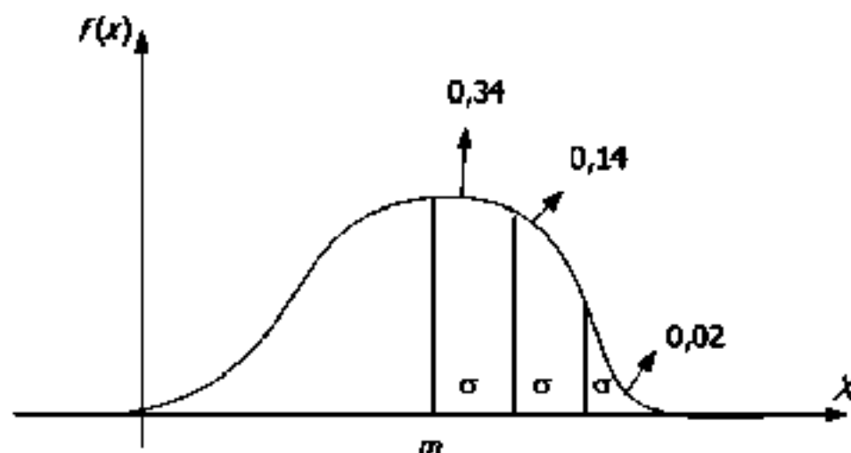
Рис. 6.3. Свойства нормального закона
