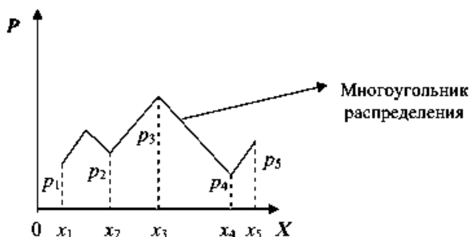
Рис. 4.1. Закон распределения дискретной случайной величины
