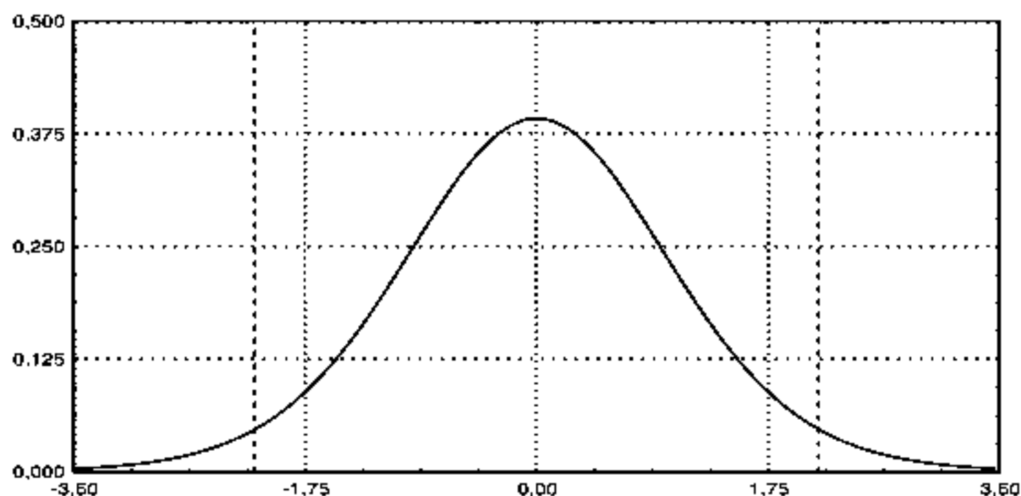
Рис. 9.2. Распределение Стьюдента ( k = 15 , \beta = 0,95 , t_{15, \alpha/2} = \pm 2,131 )
