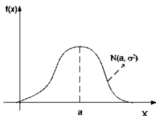
Рис. 6.1. Нормальное распределение
