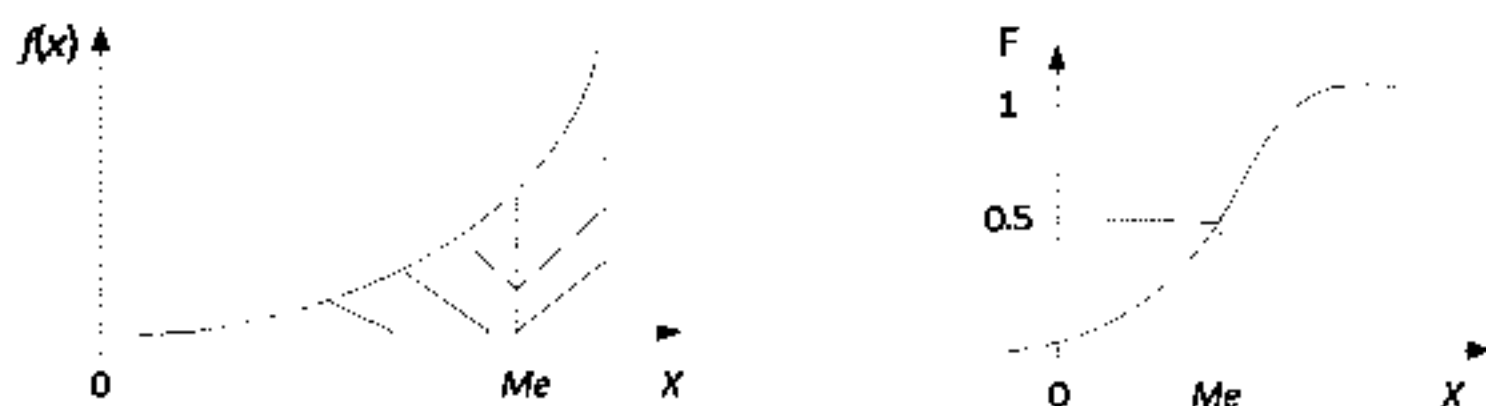
Рис. 4.6. Медиана распределения СВ
