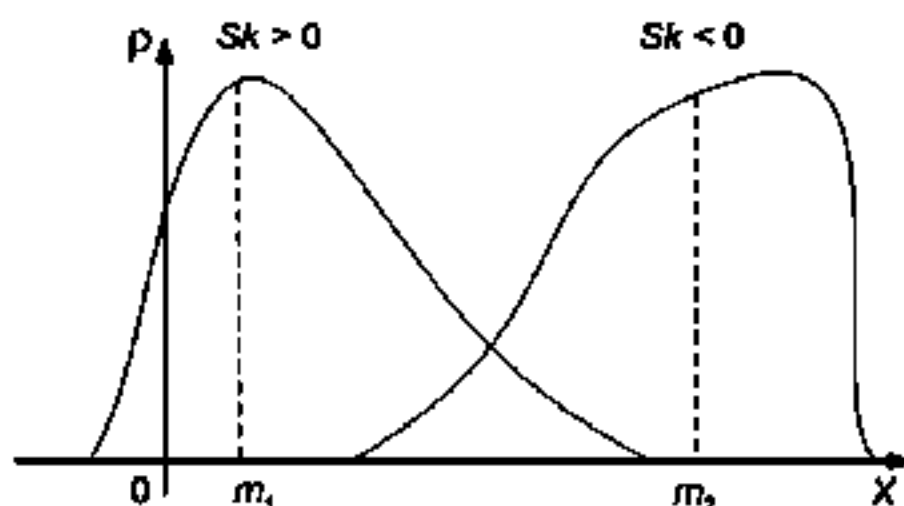
Рис. 4.7. Характеристика асимметрии распределений
