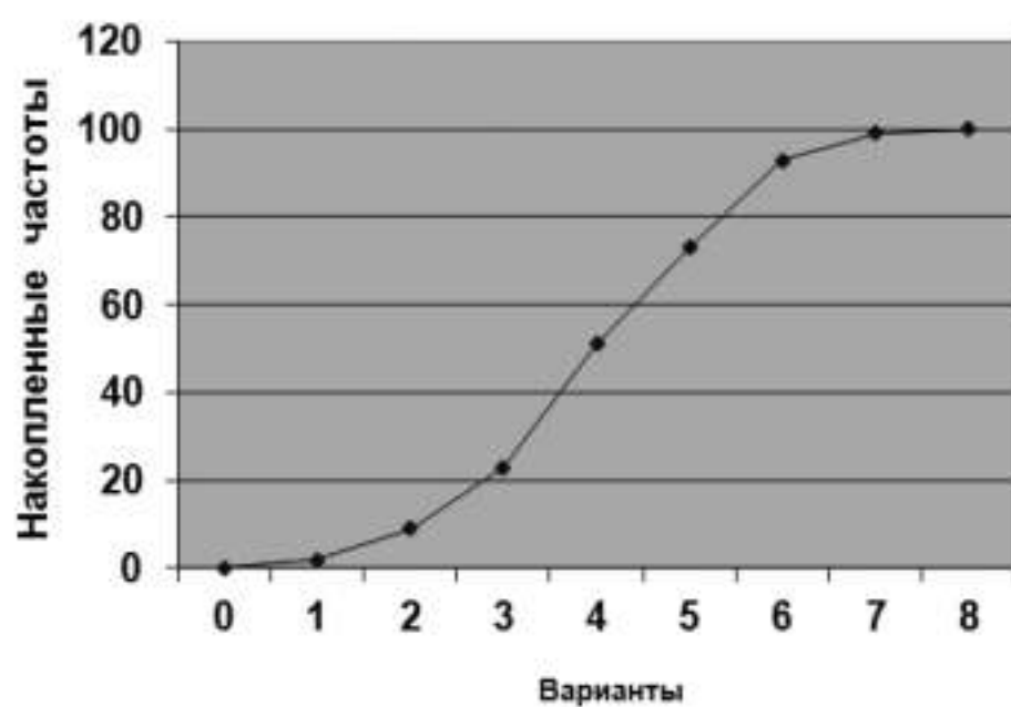
Рис. 8.3. Кумулята
