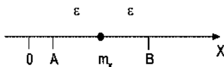
Рис. 7.1. Отрезок интегрирования
