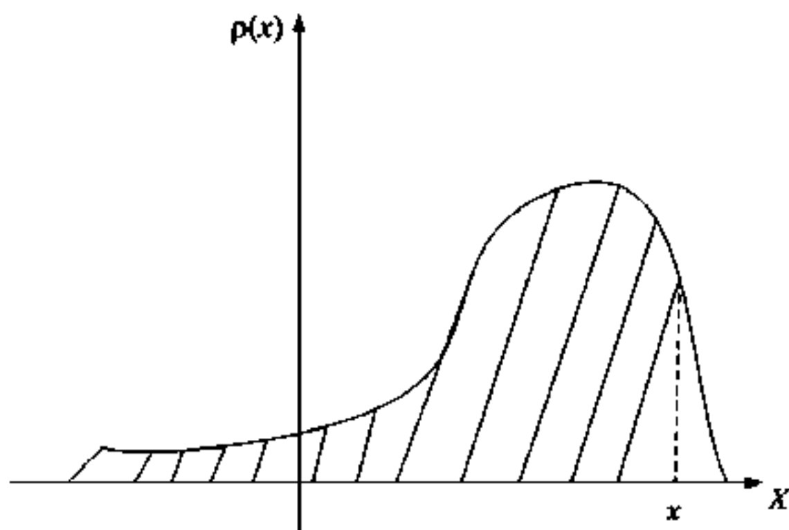
Рис. 4.4. Вычисление функции распределения через плотность СВ
