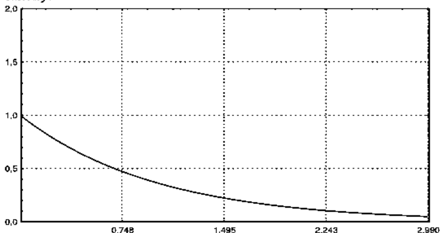
Рис. 6.5. Дифференциальная функция показательного распределения ( \lambda = 1 )
