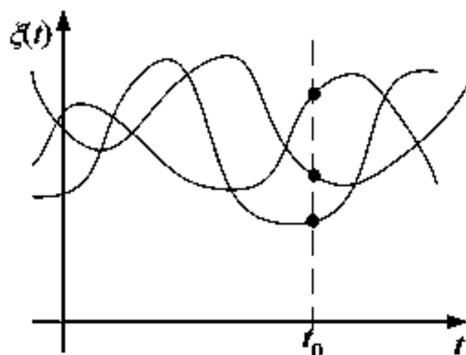
Рис. 11.1. Сечение случайного процесса
