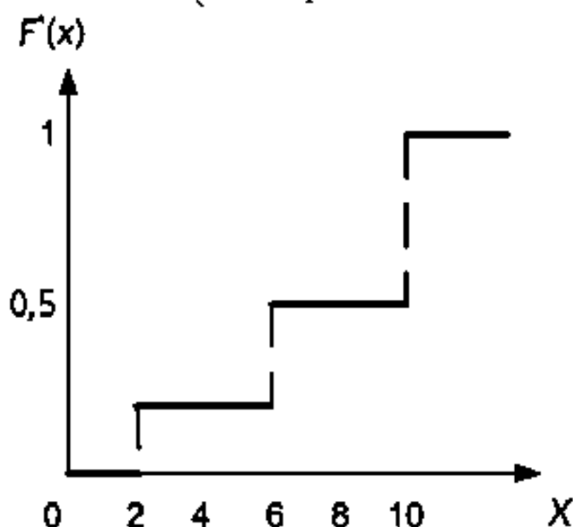
Рис. 8.4. Статистическая функция распределения (гистограмма)
