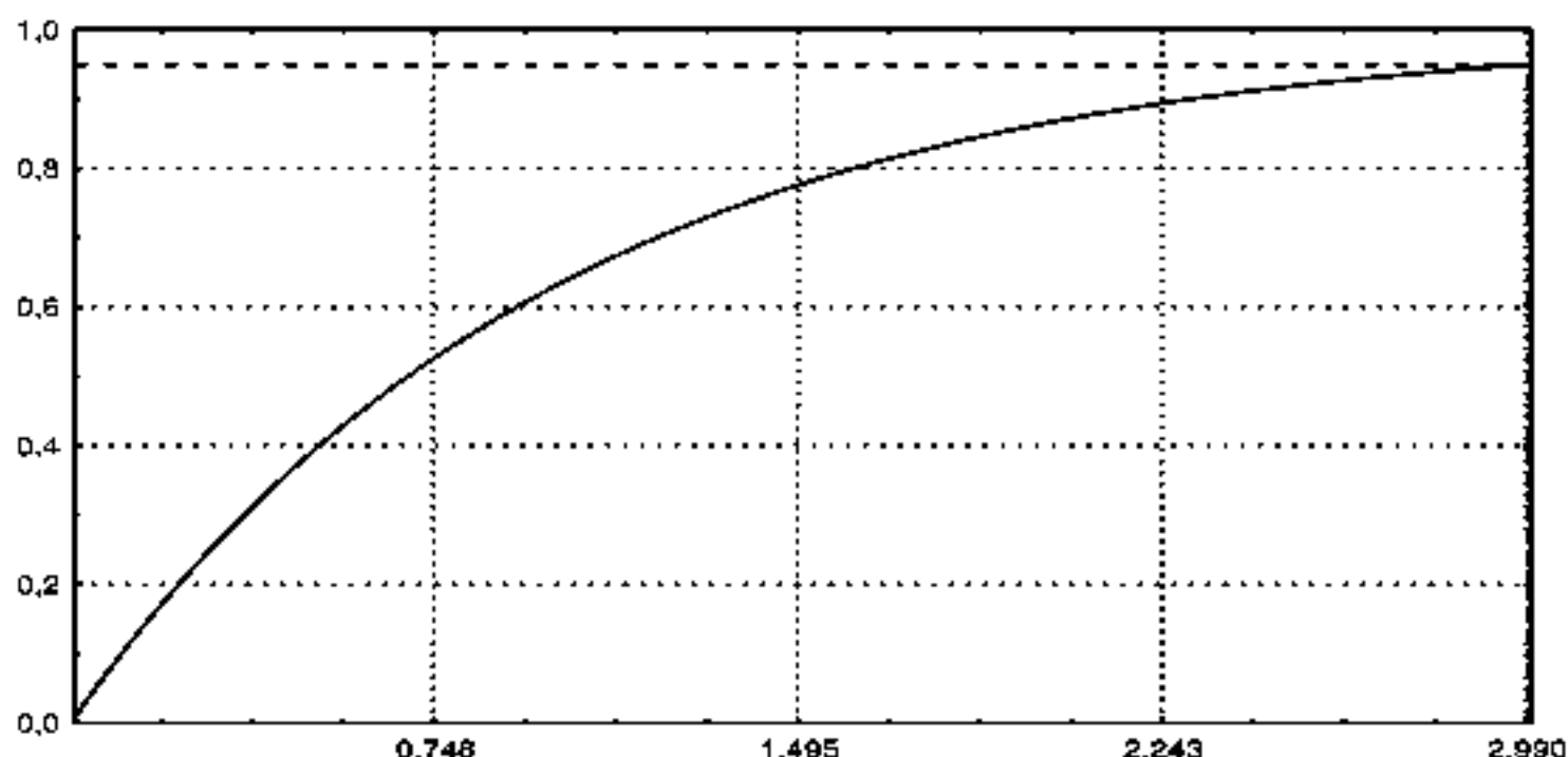
Рис. 6.6. Интегральная функция показательного распределения ( \lambda = 1 )
