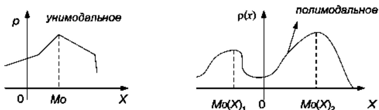
Рис. 4.5. Мода распределения СВ
