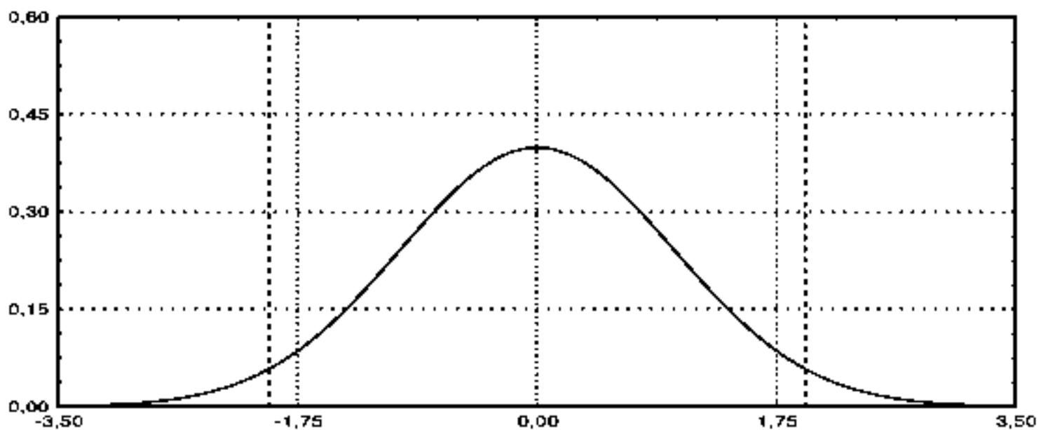
Рис. 9.1. Гауссово распределение ( N(0, 1) , \beta = 0,95 , U_{\alpha/2} = \pm 1,96 )
