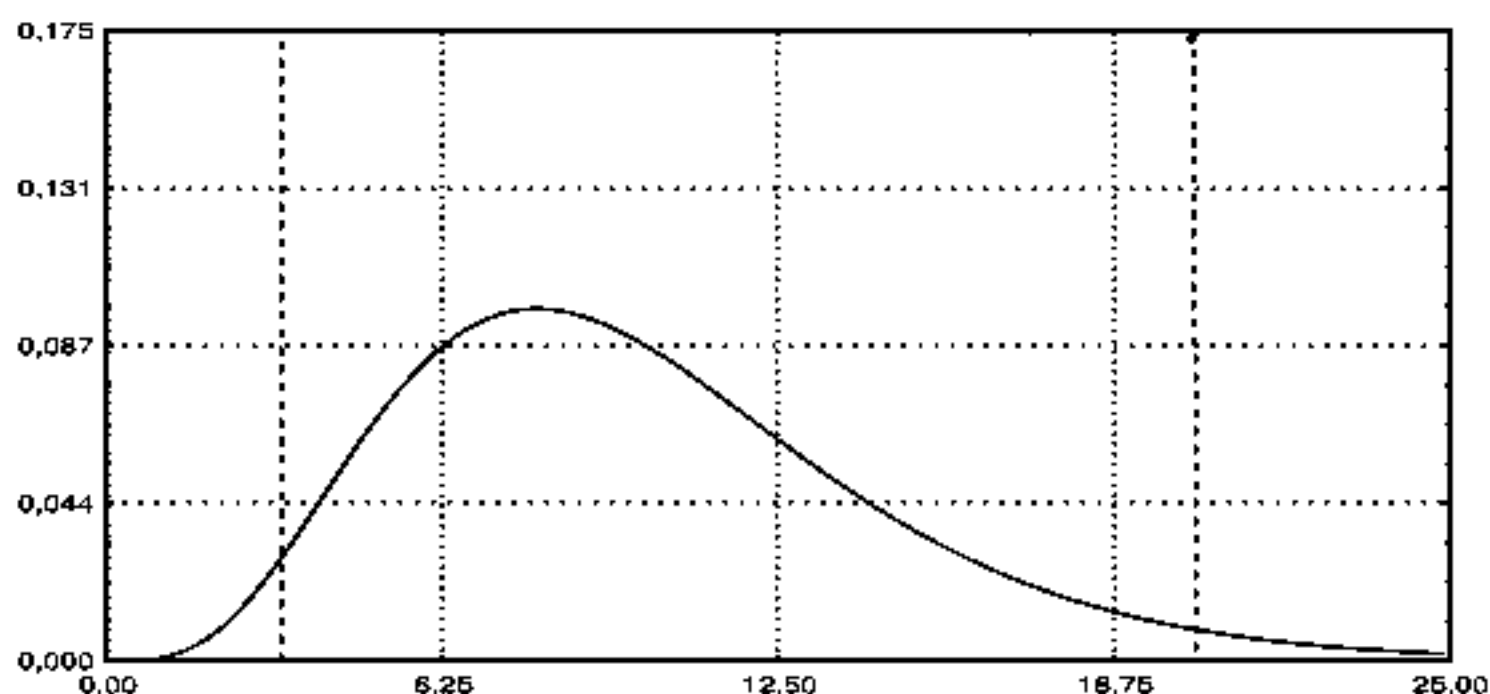
Рис. 9.3. Распределение \chi^2 ( k=10 , \beta=0,95 , \chi^2_{10;0,025}=3,247 , \chi^2_{10;0,975}=20,486 )
